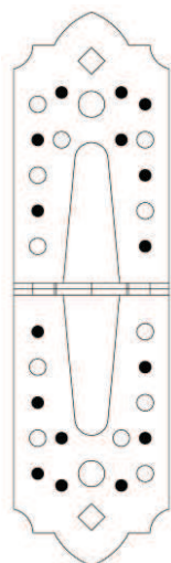
SDSKP 1
