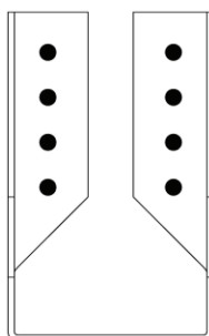
SDSWBZ 14
